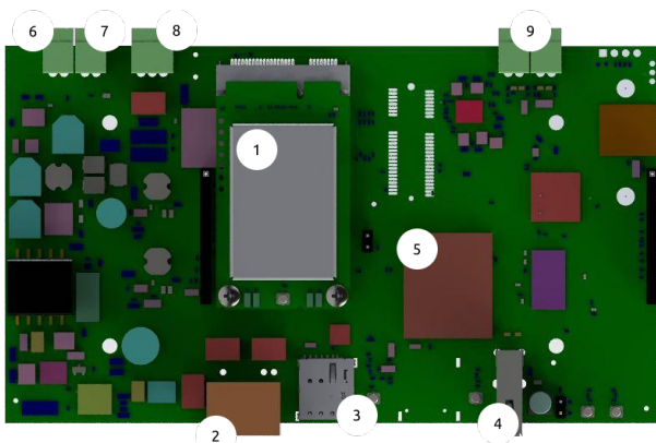
Abbildung 5: Hauptplatine
