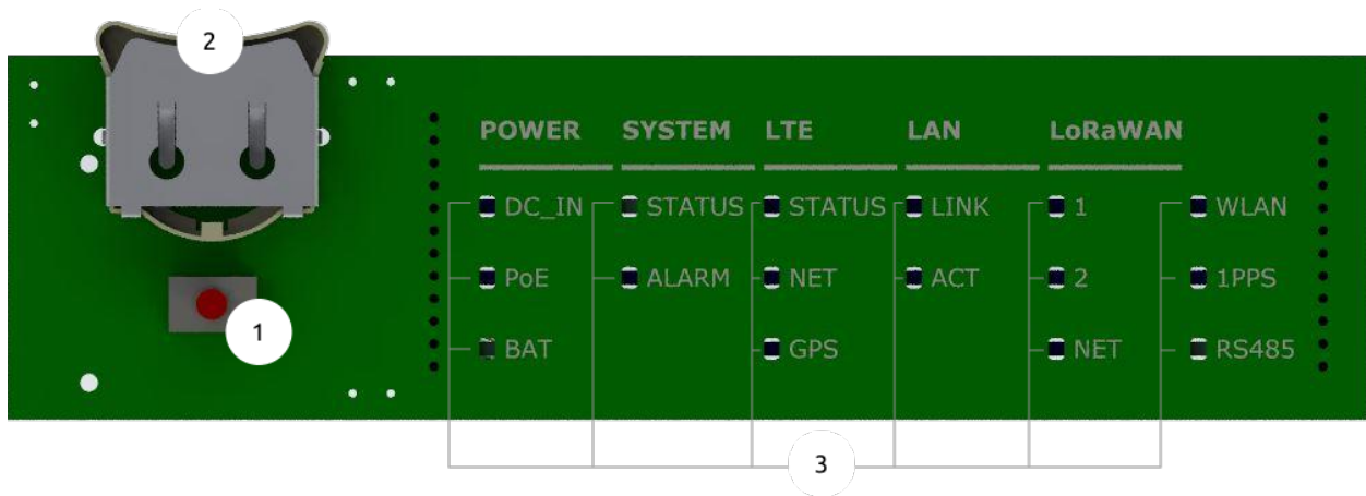
Abbildung 6: Anzeigeplatine
