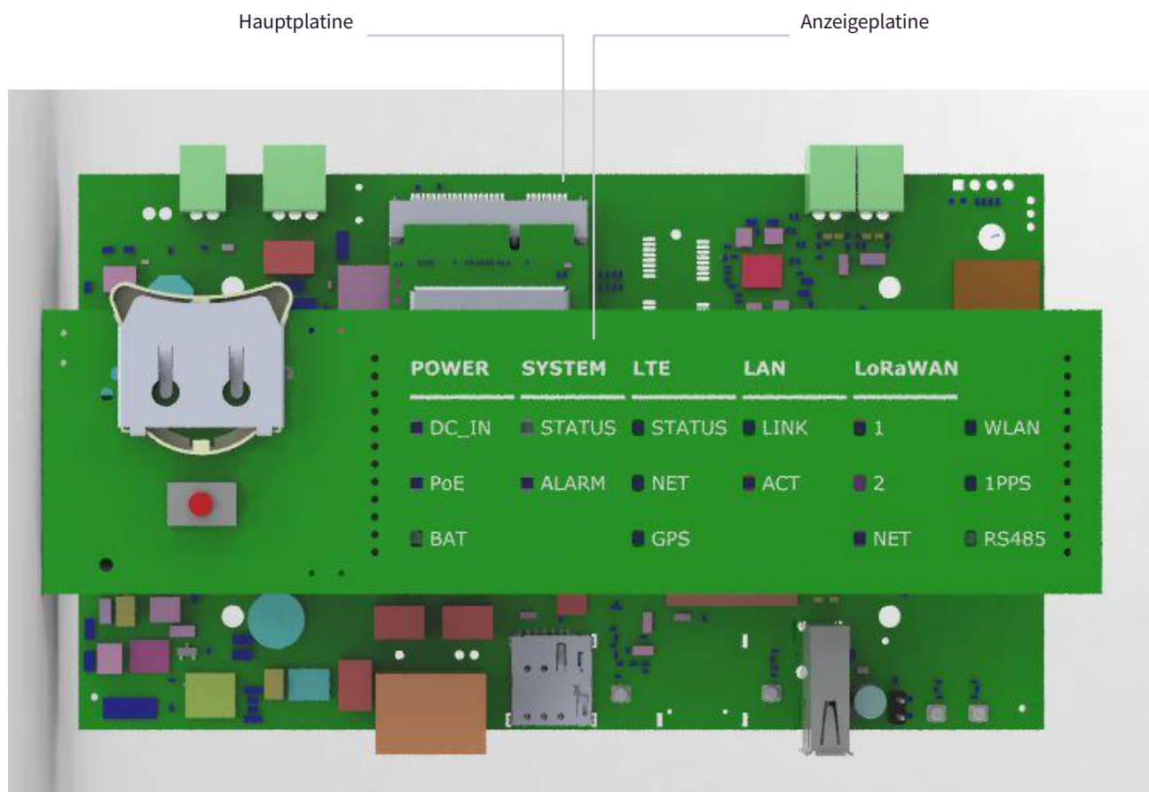
Abbildung 1: Doppelte Leiterplatte
